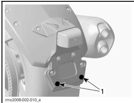
1. Eksisterende puter på feste for nummerskilt
