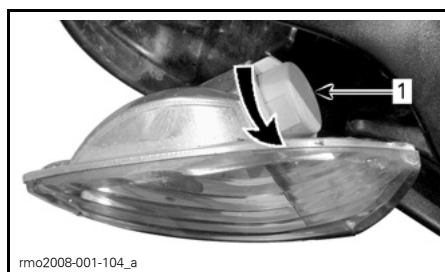
1. Kontakt for blinklys foran
