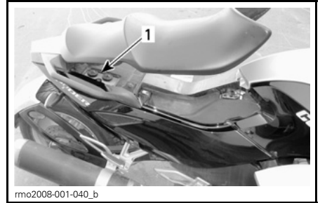
1. Bremsevæskebeholder
