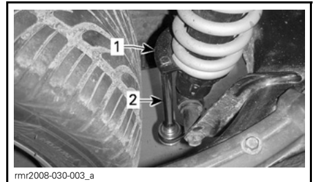
1. Nokafsteller 2. Draaisleutel met verlenging
