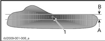
rbl2009-001-008_a LICHTBUNDEL VAN DE DIMLICHTEN OP HET TESTOPPERVLAK — LANDEN WAAR LINKS WORDT GEREDEN
