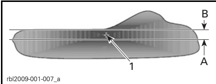
rbl2009-001-007_a LICHTBUNDEL VAN DE DIMLICHTEN OP HET TESTOPPERVLAK — LANDEN WAAR RECHTS WORDT GEREDEN
