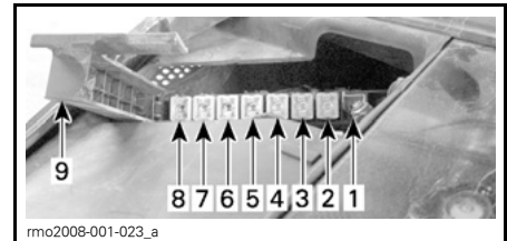
ZEKERINGEN ONDER HET ZADEL
