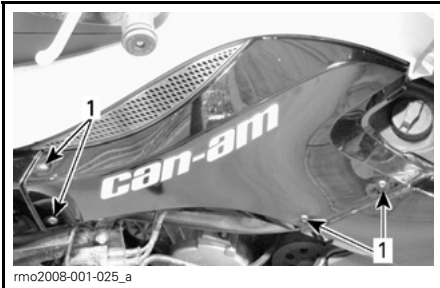
1. Torx-schroeven van het bovenste zijpaneel
