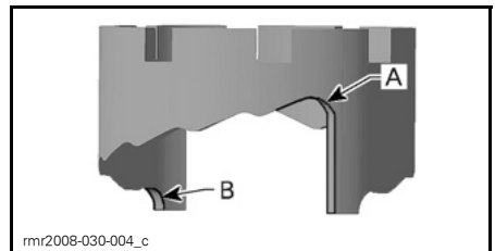
A. Zachte afstelling (stand 1) B. Harde afstelling (stand 7)
