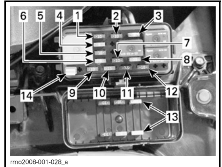
FUSIBLES SITUADOS BAJO LA CUBIERTA DE SERVICIO
