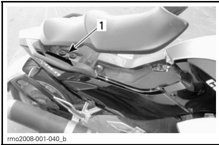
1. Depósito de líquido de frenos
