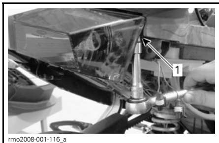
1. Extracción del tornillo Torx tras la lente
