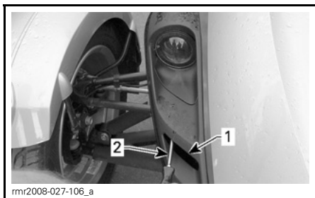
rmr2008-027-106_a 1. Conducto de aire 2. Destornillador
