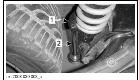
1. Ajustador de leva 2. Trinquete con extensión
