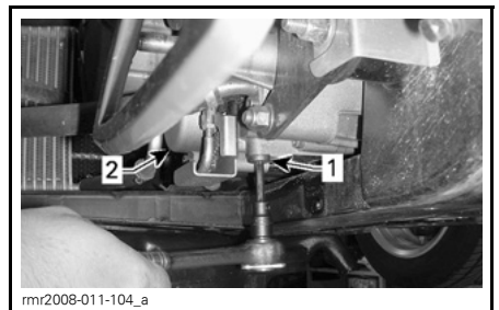
1. Tapón de drenaje de aceite del motor 2. Cubierta de filtro de aceite
