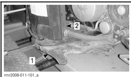
1. Placa inferior 2. Depósito de aceite
