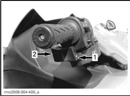
1. Upshift 2. Downshift
