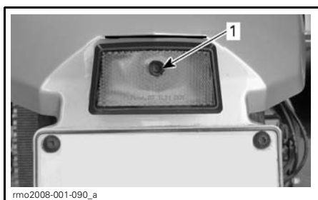
1. Vis de lentille de plaque d'immatriculation
