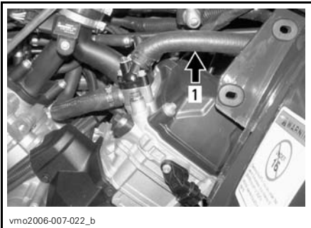
1. Hose pincher
