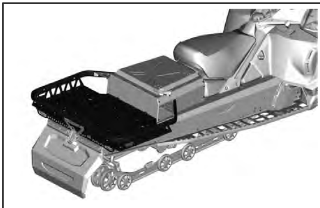
HD 机架
