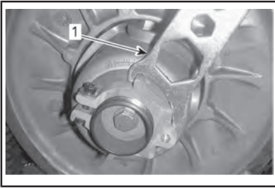
调节器轮毂
