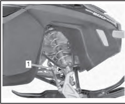
典型示例 - 凸轮型预载
