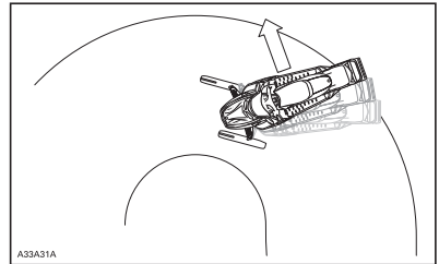
转向过度
