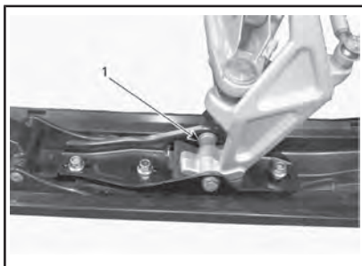
1. 间隔器在雪橇支腿内侧
