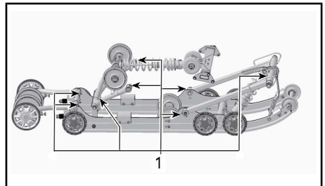
1. Schmierlager
