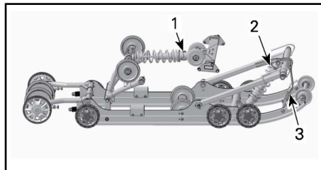
HINTERE AUFHÄNGUNG PPS-5900A UND PPS-6900A
