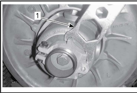
1. Aufhängungseinstellvorrichtung
