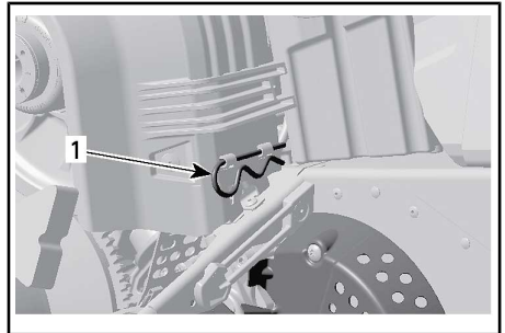
1. Arretierstift
