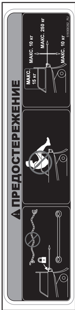
НАКЛЕЙКА 10 – МОДЕЛИ 49 Ranger
