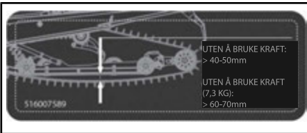
DEKAL 6 – PÅ 49 RANGER
