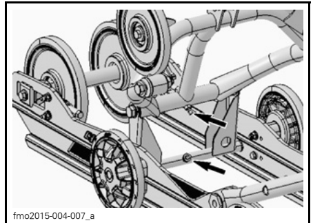
TYPBILD PPS2-SMÖRJNIPPLAR (BAK)
