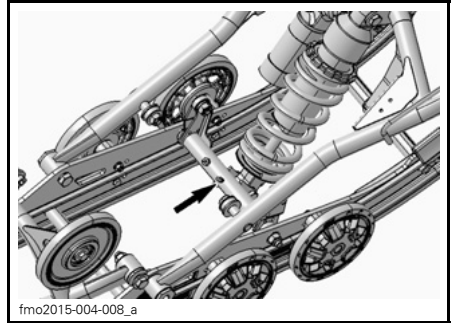
TYPBILD PPS2-SMÖRJNIPPLAR (FRAM)
