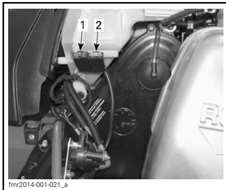
HÖGER SIDA AV MOTORRUMMET 1. Laddningssäkring 2. START/REVERSE-säkring
