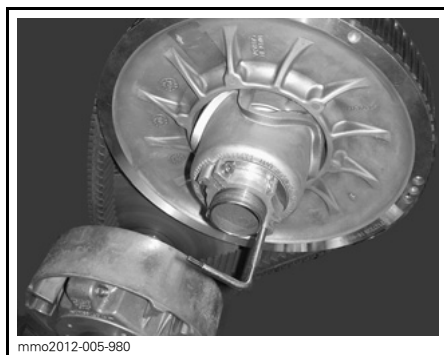
DISPOSITIVO DI ESPANSIONE DELLA PULEGGIA INSTALLATO SUL MOZZO DEL REGISTRO.
