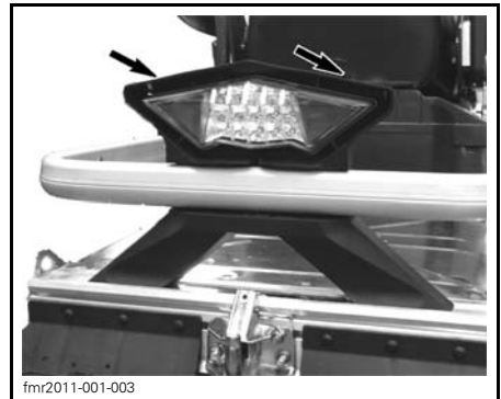
ESTRARRE LA LAMPADINA E SOSTITUIRLA
