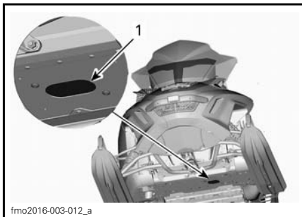
1. Tyhjennystulppien peitekansi
