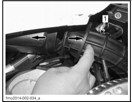
1. Luftintagsrör
