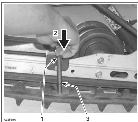
BANDSPÄNNINGSTESTARE
