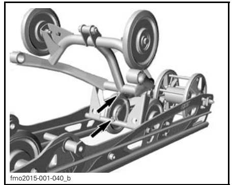
TYPBILD PPS2 3700 OCH 3900-SMÖRJNIPPLAR (BAK)
