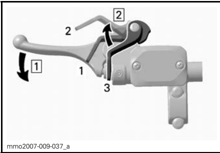
TYPBILD — AKTIVERA BROMSEN Step 1: Steg 1: Håll in bromshandtaget Step 2: Steg 2: Justera låsspaken
