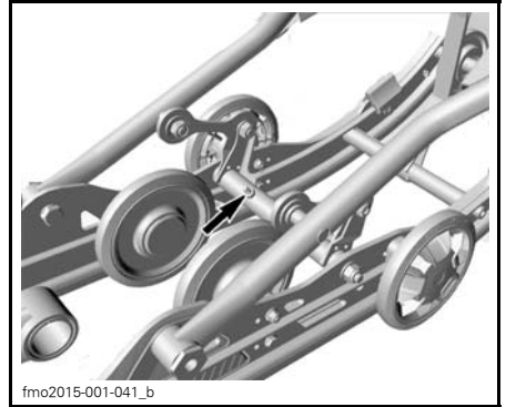
TYPBILD PPS2 3700 OCH 3900-SMÖRJNIPPLAR (FRAM)
