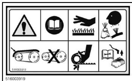
ON PROTEZIONE DELLA PULEGGIA - ETICHETTA 7
