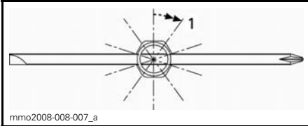
CANDELA USATA 1. Serrare di 1/10 di giro
