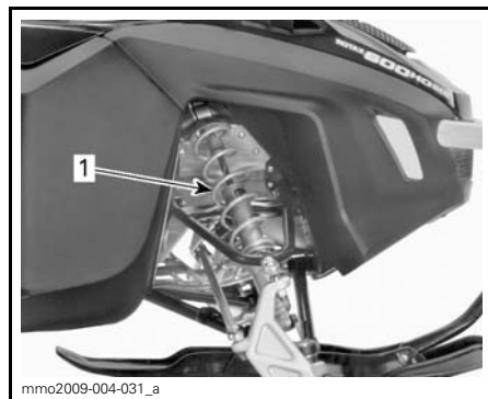
TIPICO - SOSPENSIONI ANTERIORI
