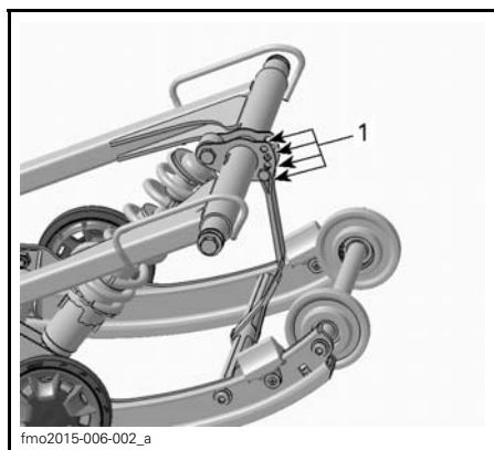
TIPICO 1. Regolazione dei fori (cinghia di fermo)
