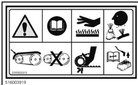
SULLA PROTEZIONE DELLA PULEGGIA - ETICHETTA 8
