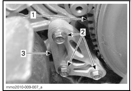
1. Puleggia motrice 2. Viti del fermo motore 3. Fermo motore
