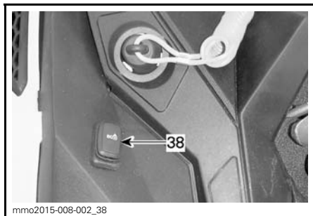
TIPICO - LATO SINISTRO DEL SERBATOIO - SOLO ACE 900
