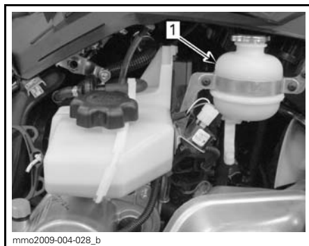
1. Linea di livello freddo
