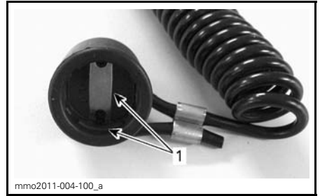
ESTREMITÀ DEL CORDONCINO DI SICUREZZA
