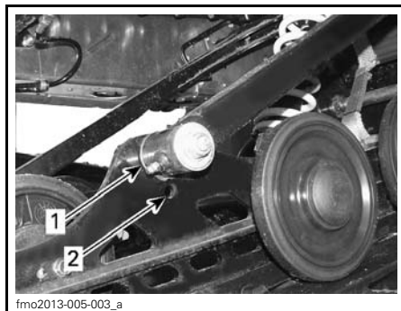
BRACCIO CENTRALE
