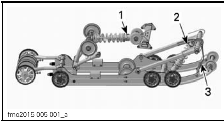
HINTERE AUFHÄNGUNG PPS-5900A
