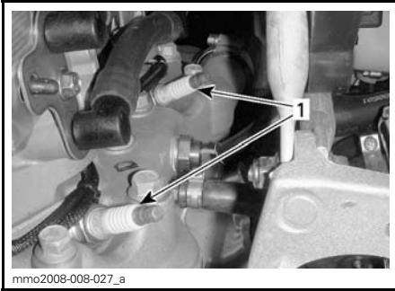
LINKE SEITE DES MOTORRAUMS 1. Zündkerzen
