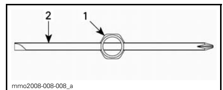
DRAUFSICHT 1. 16-mm-Buchse 2. Schraubendreherstange
