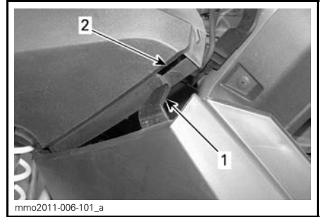
1. Linguetta del pannello laterale inferiore 2. Scanalatura della carenatura del fondo
