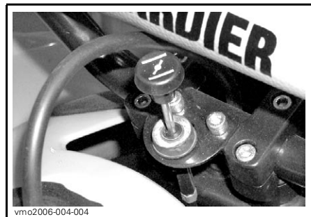
ÉTRANGLEUR OUVERT
