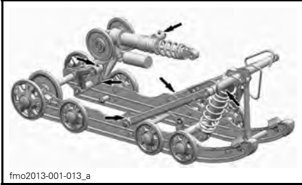
1. TYPBILD PPS-smörjniplor
