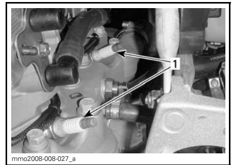
VENSTRE SIDE AV MOTORROMMET 1. Tennplugg
