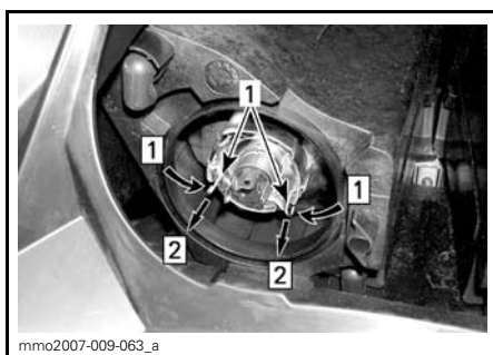
Fase 1: premere su entrambi i lati Fase 2: tirare per rilasciare
