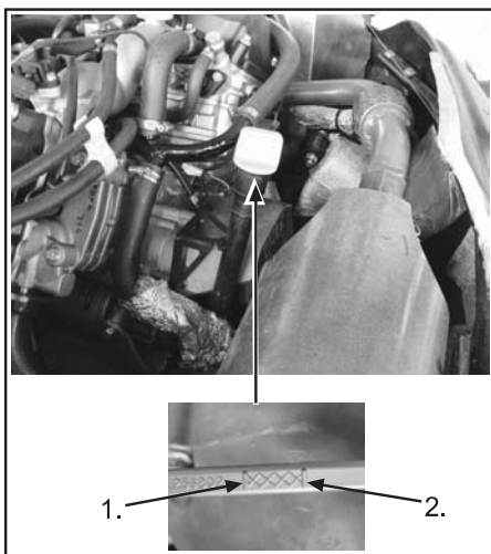
PRO V-800-RESERVETANK VED EKSOSPOTTEN
