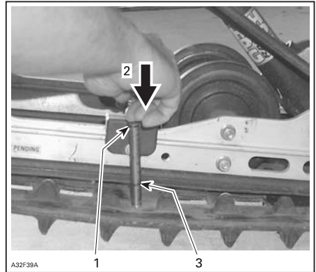
RIEMENSpannungsprüfgerät
