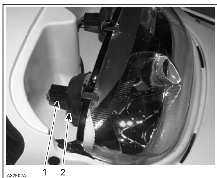
1. Glühlampenanschluss 2. Gummikappe
