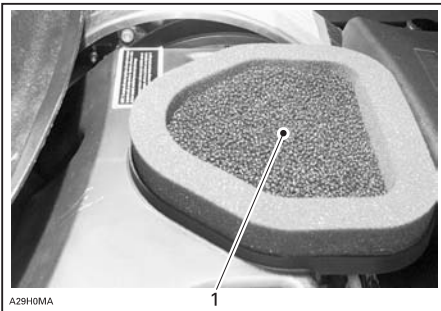
1. Sekundär-Luftfilter
