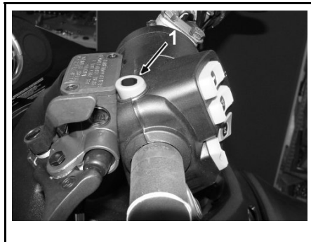
1. Taste für elektrische Hupe
