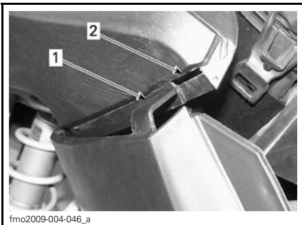
1. Tab 2. Slot
