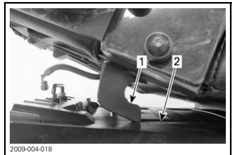
1. Sitzhaken 2. Aussparung
