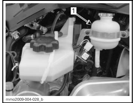
1. Kühlmitteltank
