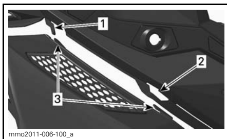
1. Konsolenhaken 2. Konsolenschlitz 3. Mittlere Rastungen der Verkleidung
