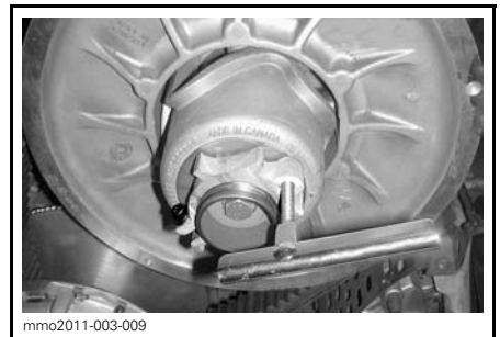
RIEMENSCHLEIBEN-ERWEITERUNG AN DER ALUMINIUM-EINSTELLERNABE
