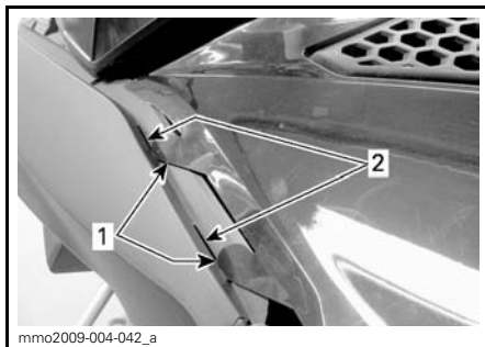
1. Laschen 2. Aussparungen
