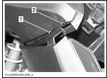
1. Lasche 2. Aussparung
