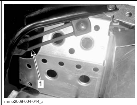
1. Gummizugelement
