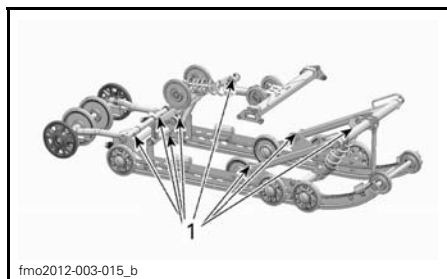
1. Lage der Schmiernippel
