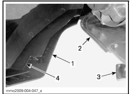
1. Unterer Bereich 2. Aluminiumfahrgestell 3. Aluminiumlasche 4. Aussparung für die Abdeckung
