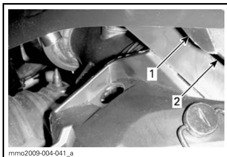
1. Lasche 2. Aussparung
