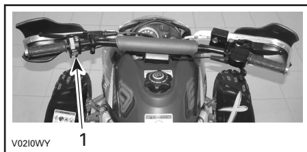
1. Interrupteur multifonctionnel
