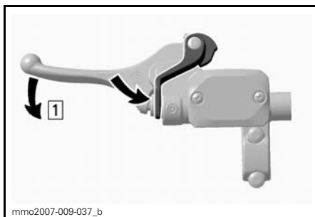
TYPEBILDE – FRIGJØRINGSMEKANISME
