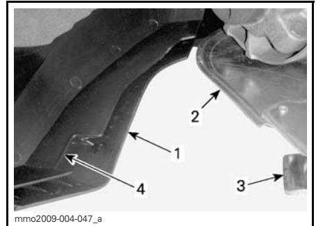
1. Partie inférieure 2. Châssis en aluminium 3. Languette en aluminium 4. Encoche du flanc
