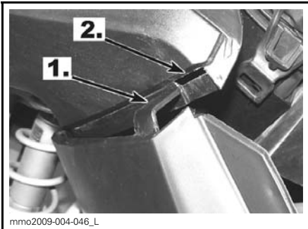
1. Languette 2. Encoche
