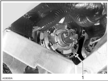
1. Anneau de verrouillage
