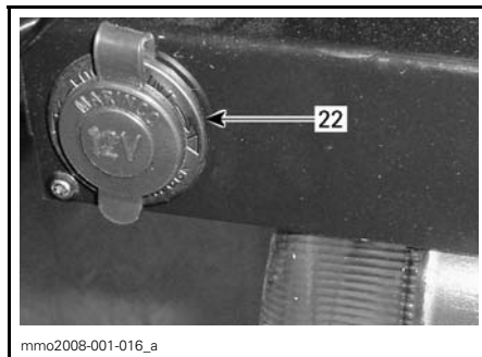
mmo2008-001-016_a UNIQUEMENT MODÈLE YETI PRO V-800 — PORTE-BAGAGES ARRIÈRE
