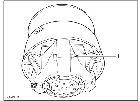
1. Desserrez seulement assez pour permettre la rotation de la vis d'étalonnage
