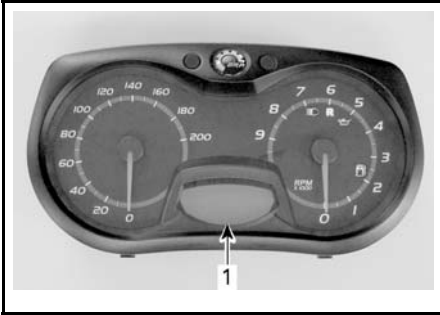
ANALOGINEN/DIGITAALINEN MITTARI
