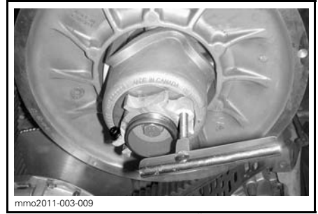
II-VARIAATTORIN AVAUSTYÖKALU ALUMIINIINENSÄ SÄÄTIMEN NAVASSA
