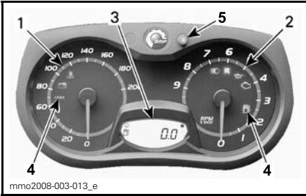
ANALOGINEN/DIGITAALINEN MITTARI
