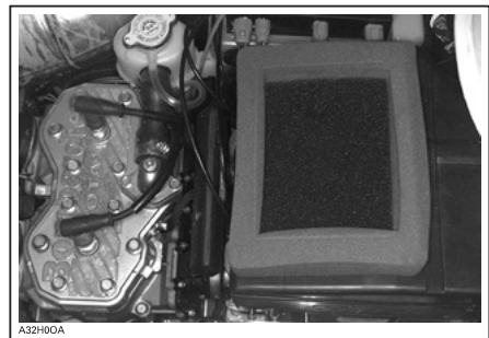
1. Sekundært luftfilter
