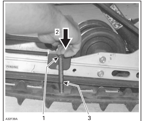
BELTESTRAMNINGSTESTER
