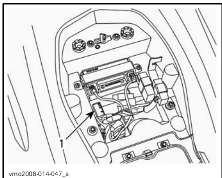
1. Porte-fusible
