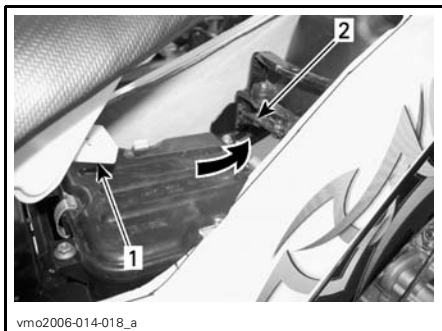
1. Languette 2. Crochet
