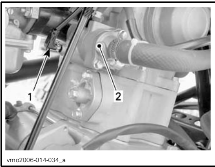
1. Sonde de température 2. Logement de thermostat
