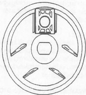
Kuva 1 Bild 1 Picture 1 Painolohkojen asema Vikblocken position Position of weights
