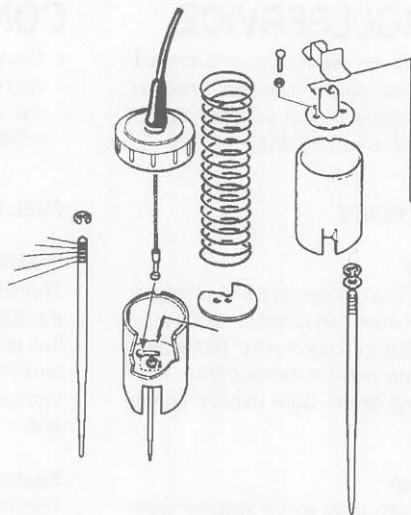
Kaasuviijerin irroitus Losstagnig av gasviajer Gas wire, loosening
