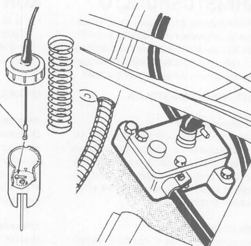
Polttoainepumppu Bränslepump Fuel pump
