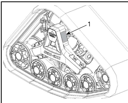
TYYPILLINEN - APACHE 360 -TELAKO- KOONPANO
