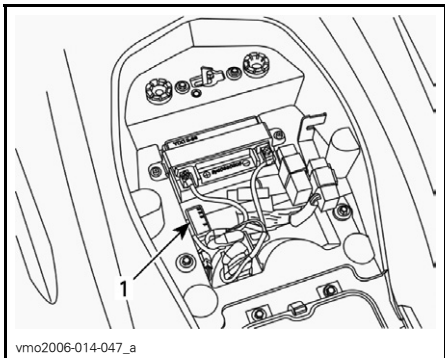
1. Zekeringhouder
