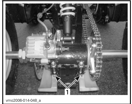
1. Borgbouten kettingspanner
