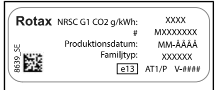
TYPBILD - NRMM-IDENTIFIERINGSDEKAL
