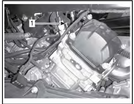
1. Främre cylinderns luftningsskruv
