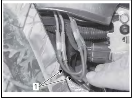
1. Fusibili
