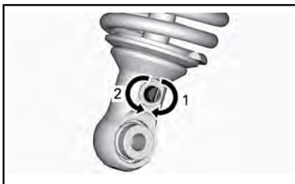
SMORZAMENTO IN ESTENSIONE - PARTE INFERIORE DELL'AMMORTIZZATORE
