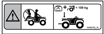
LABEL 4: OUTLANDER X mr (570): ACHTERS PATBORD (RAADPLEEG DE SPECIFICATIES VOOR WAARDEN)
