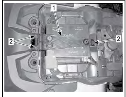
1. Accuhouder 2. Borgschroeven
