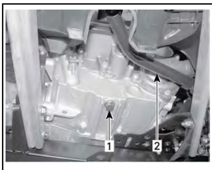
1. Oliefilterdeksel
