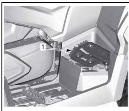
1. Voetsteun voor rijden door de modder
