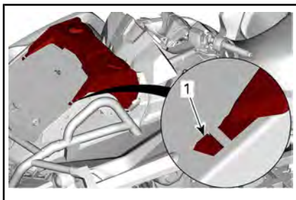
1. Afdektab
