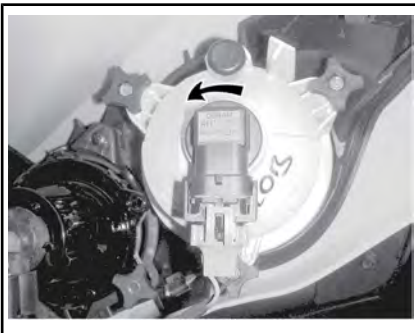
BINNENKANT VOORZIJDE SPATBORD
