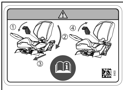
HINWEISSCHILD 10 - UNTER DEM BEIFAHRERSITZ
