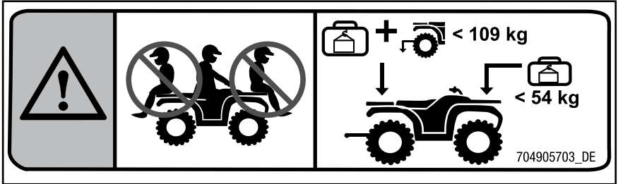
HINWEISSCHILD 5
