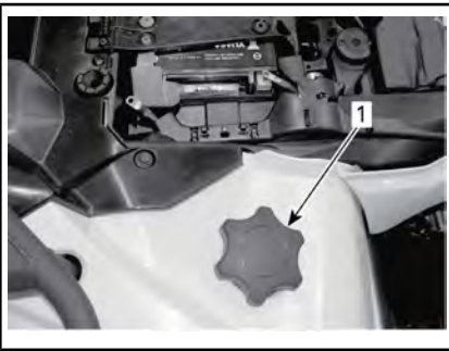
1. Kraftstoffbehälterkappe
