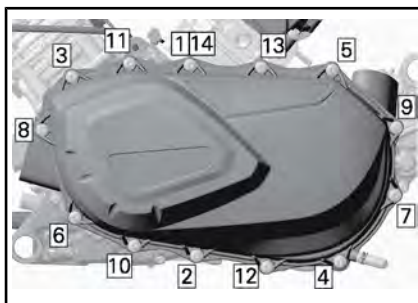
CVT-ABDECKUNG-ANZUGSREIHENFOLGE
