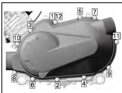
CVT-ABDECKUNG-ANZUGSREIHENFOLGE
