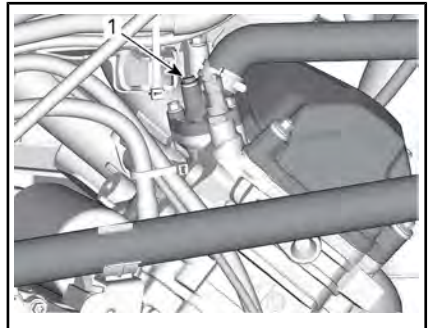
1. Entlüftungsschraube des vorderen Zylinders
