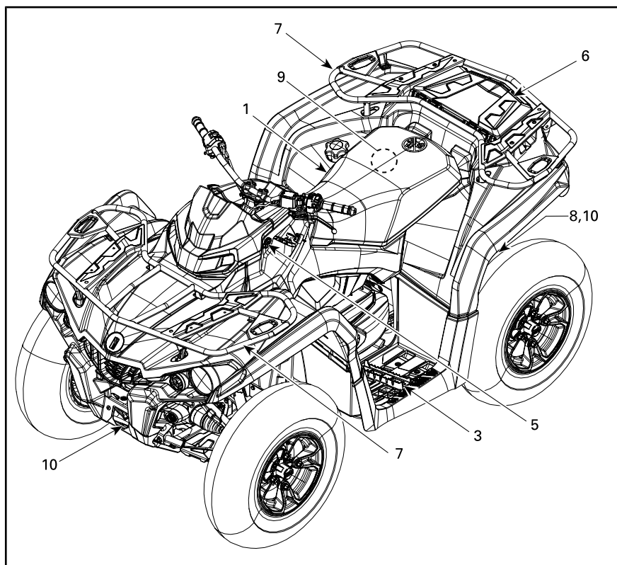
TYPISCH – EINSITZER-MODELLE
