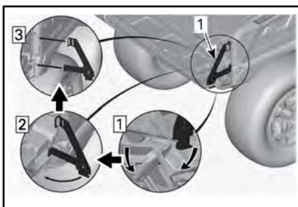
1. Höger stödkonsol
