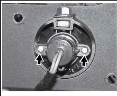
SKRUVA LOSS HÅLLSKRUVARNA FRÅN DEN BAKRE RIKTNINGSVISARGLÖDLAMPAN
