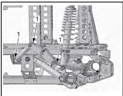
KRÄNGNINGSHÄMMARE
