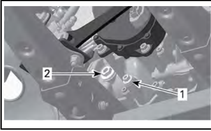
TYPBILD - 650-MOTOR
