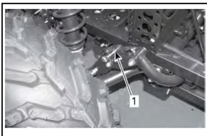
1. Spärrad krängningshämmarsprint
