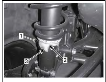
FJÄDRINGENS JUSTERINGSVERKTYG
