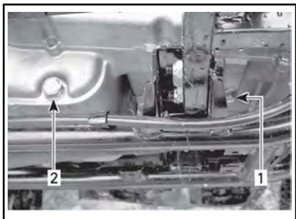
TAPÓN DE DRENAJE — LADO IZQUIERDO DEL MOTOR
