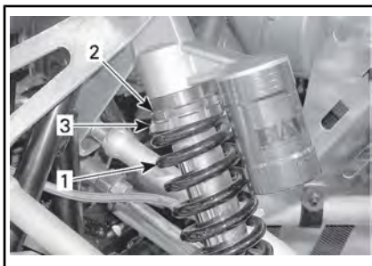
DS 90 X, SUSPENSIÓN DELANTERA
