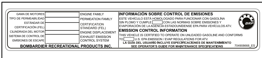
TÍPICO - UBICACIÓN: DEBAJO DEL GUARDABARROS TRASERO
