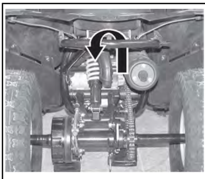
TODOS LOS MODELOS — PUNTO DE ANCLAJE TRASERO
