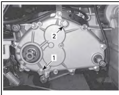
1. Bouchon de vidange de boîte de vitesses
