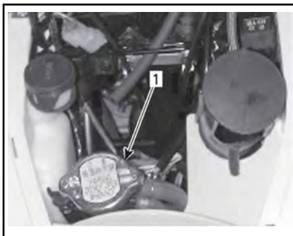
1. Bouchon du radiateur
