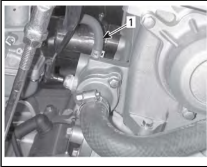
1. Flexible de dérivation
