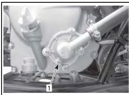
1. Bouchon de vidange du système de refroidissement
