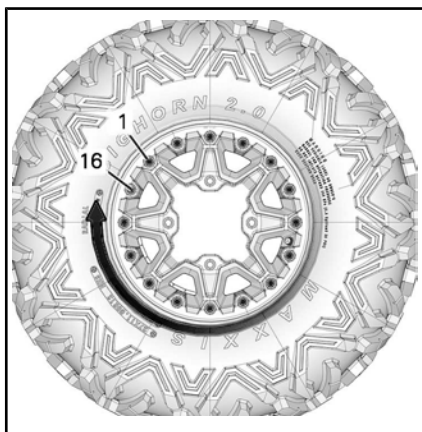
TYPISCH – ENDGÜLTIGE ANZIEHREIHENFOLGE
