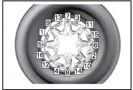
TYPISCH – ANZIEHREIHENFOLGE
