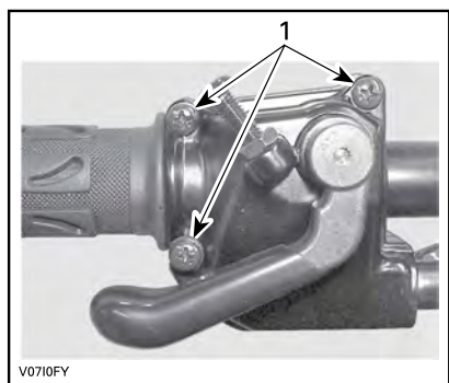
1. Diese Schrauben entfernen
