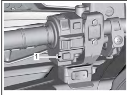
1. Override-/DPS-Taste
