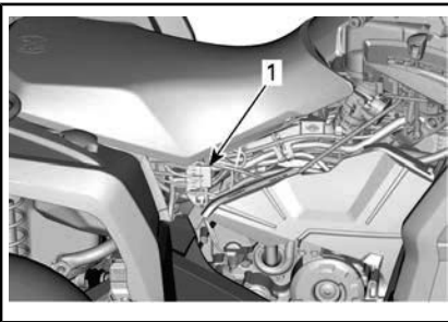
1. Collegamenti ai fusibili e ai portafusibili posteriori
