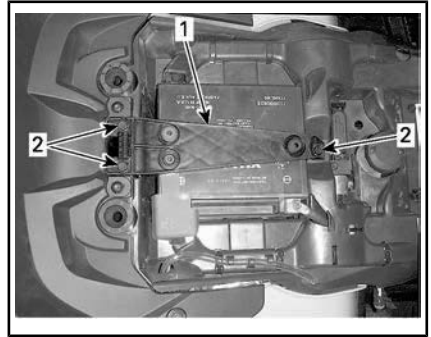
1. Porta batteria 2. Viti di blocco
