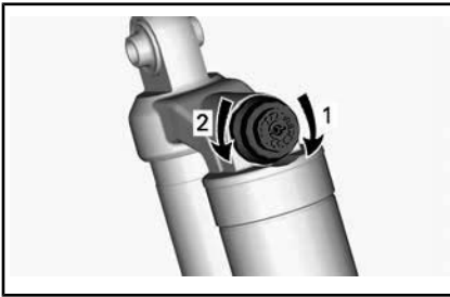
SMORZAMENTO IN COMPRESSIONE - PARTE SUPERIORE DELL'AMMORTIZZATORE
