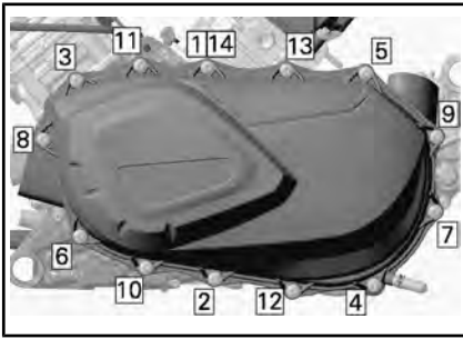
CVT-KÅPANS ÅTDRAGSSEKVENNS
