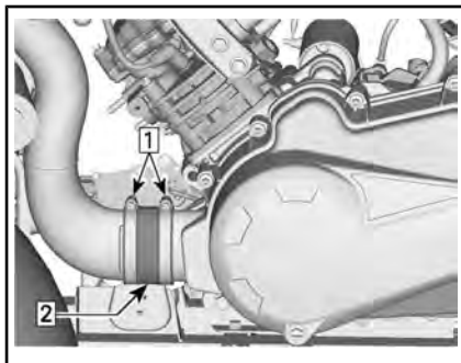
CVT-LUCHTINLAATKANAAL VERWIJDEREN
