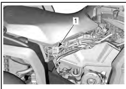
1. Porte-fusibles arrière et éléments fusibles
